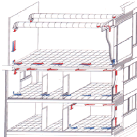
Figura 4. Spaccato assometrico del corpo B che evidenzia il sistema di circolazione dell'aria.
