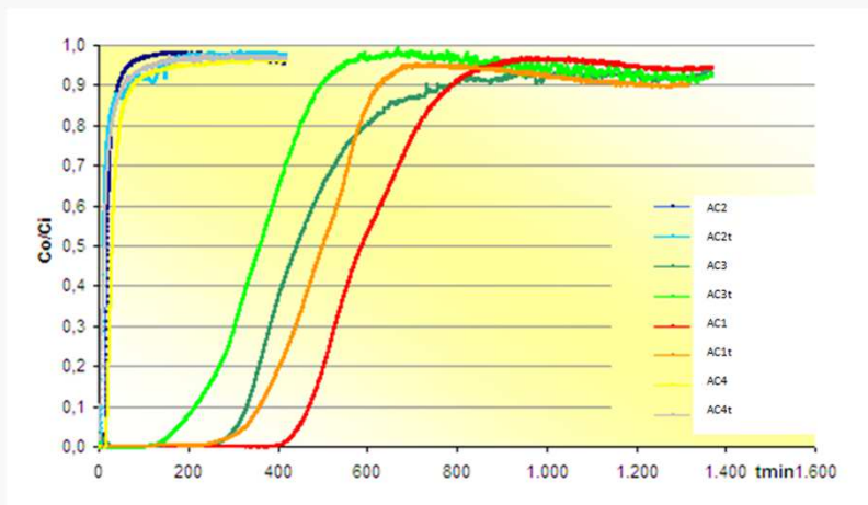
CURVE DI ROTTURA (SATURAZIONE CARBONI)
