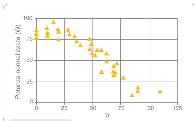
Figura 5 Potenza normalizzata verso l'angolo di incidenza
