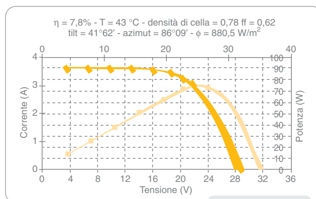
Figura 6 Caratteristiche elettriche del con celle Ersol Rainbow 3
