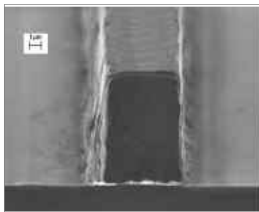
A sinistra la cella a concentrazione PhoCUS in silicio cristallino. A destra, una immagine della sezione di un finger della griglia di contatto frontale, ottenuta al microscopio elettronico a scansione. Di particolare rilevanza l'aspect-ratio del pattern fotolitografato con la tecnica lift-off in un singolo step.
