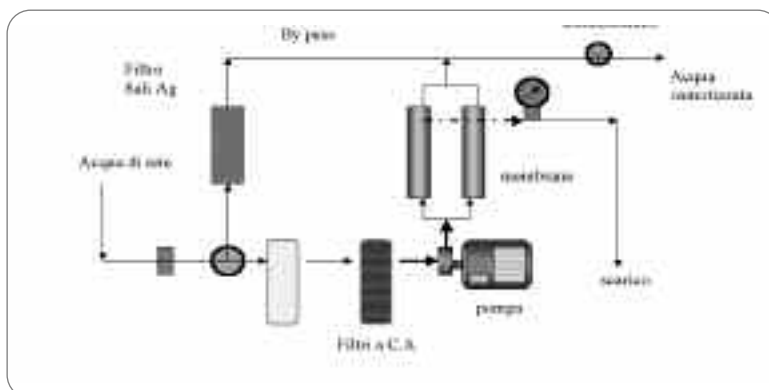
Figura 4 Schema idraulico di un depuratore d'acqua per uso domestico
