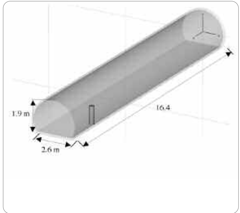
Figura 3 Modello numerico della cabina passeggeri con una sorgente e un simulatore dielettrico di passeggero
