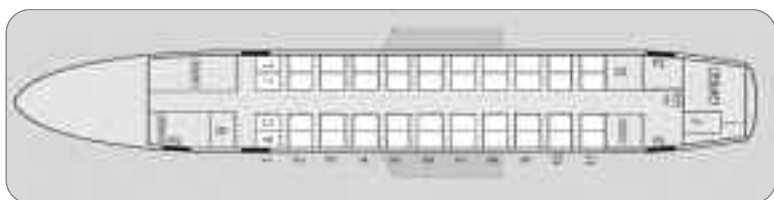
Figura 2b Sezione orizzontale/longitudinale di un ATR42 con sedili passeggeri (D: porta, G: cucina, T: toeletta, C: guardaroba)
