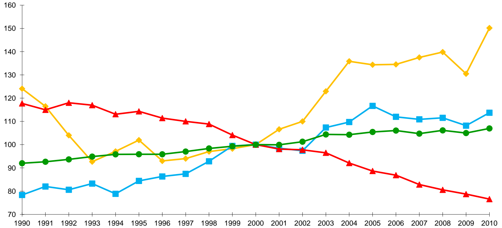
Intensità energetica per fonti - numeri indici 2000 = 100
